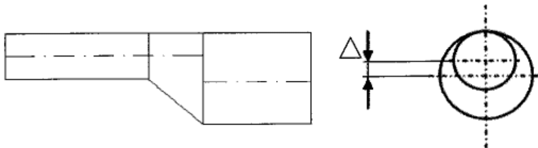
Устройство несоосного перехода труб
