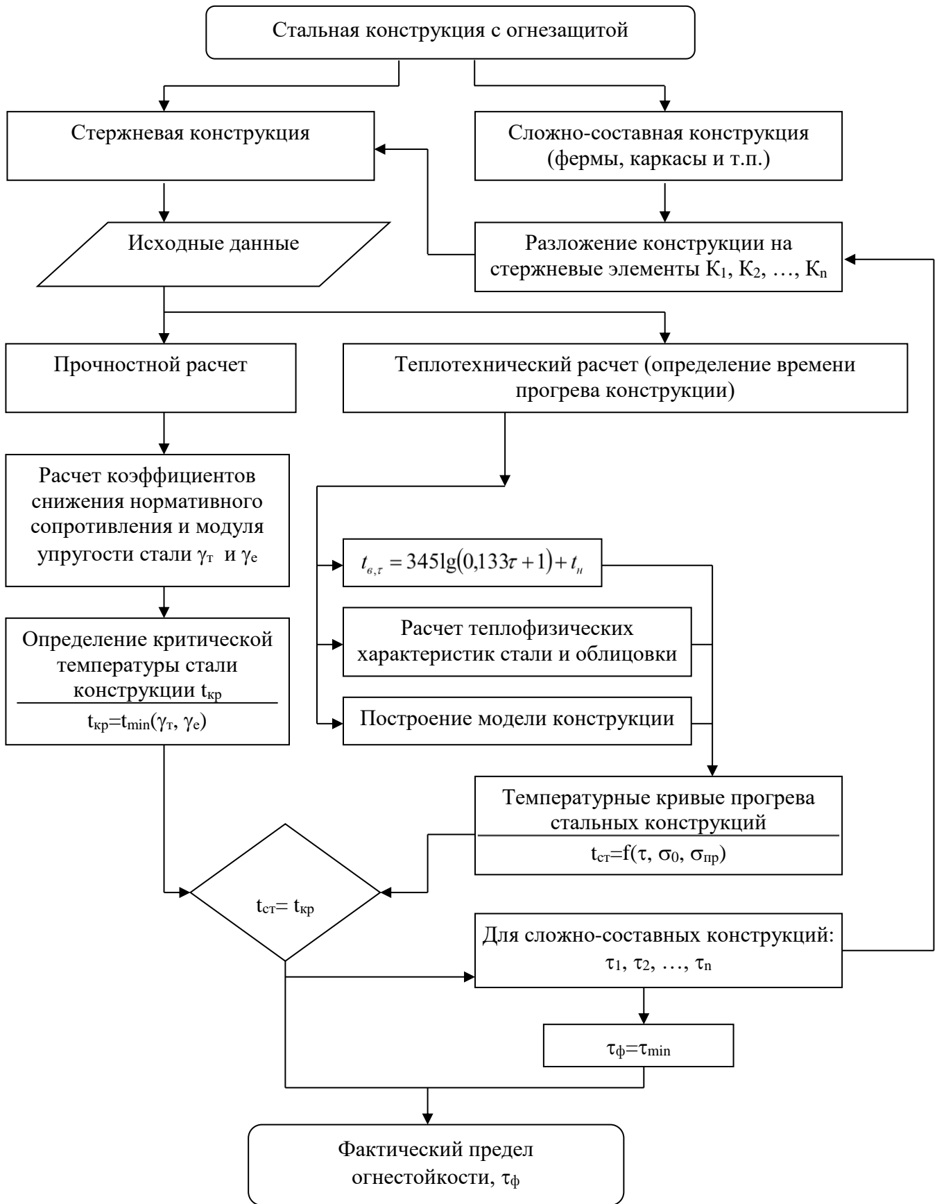
Рис. 3.1. Алгоритм определения фактических пределов огнестойкости стальных конструкций по несущей способности.
